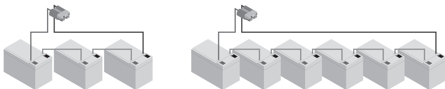
Рисунок 5. Подготовка внешних АКБ
