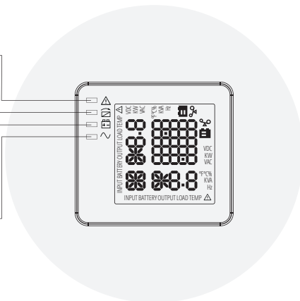
Рисунок 4. Панель управления ИБП
